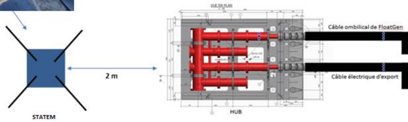
FIGURE 23 : SCHEMA ET PHOTOGRAPHIE DU DISPOSITIF STATEM (MAPPEM GEOPHYSICS, 2019).
