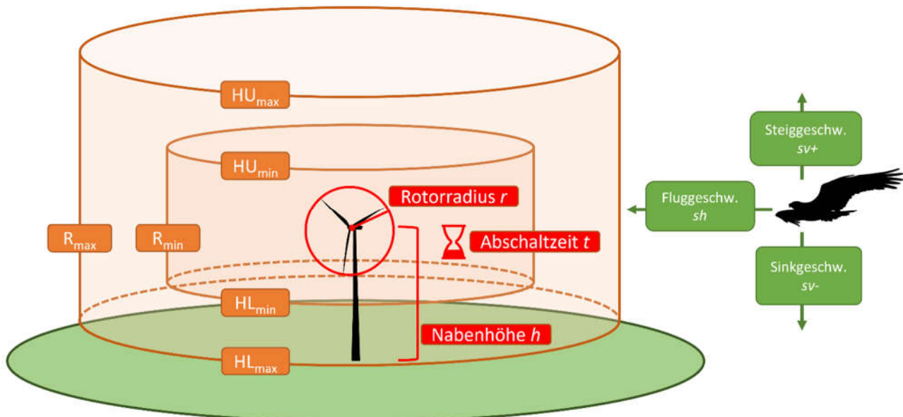
Abbildung 57: Schema zur Dimensionierung der angehobenen inneren und äußeren Abstandszylinder HU_{max} bzw. HL_{max} = obere („upper“) und untere („lower“) Begrenzung des äußeren Abstandszylinders, HU_{min} bzw. HL_{min} = obere („upper“) und untere („lower“) Begrenzung des inneren Abstandszylinders; R_{max} = Radius des äußeren Abstandszylinders, R_{min} = Radius des inneren Abstandszylinders.
