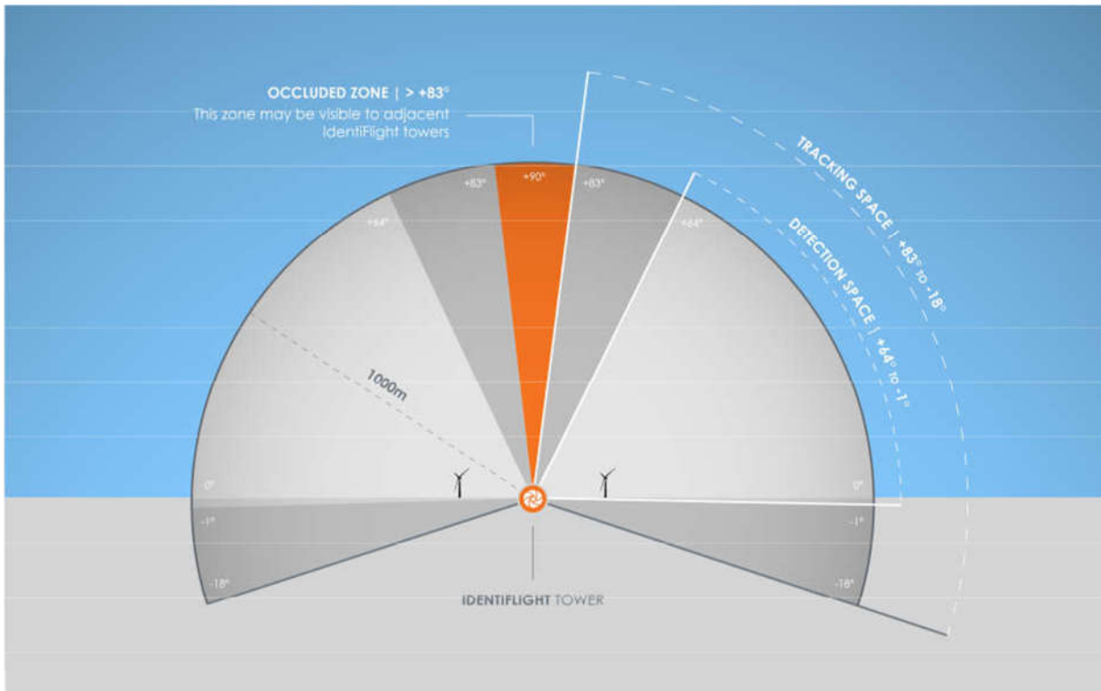
Abbildung 10: Sichtfeld eines IdentiFlight-Systems PTU V2. Quelle: Abbildung des Herstellers.
