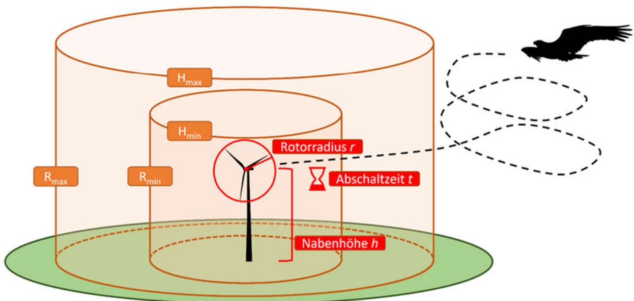
Abbildung 13: Schema zur Dimensionierung der inneren und äußeren Abstandszylinder.
