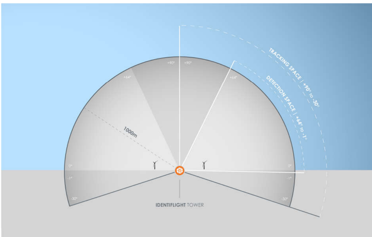
Abbildung 11: Sichtfeld eines IdentiFlight-Systems PTU V3. Quelle: Abbildung des Herstellers.
